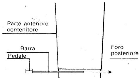
Figura C Impugnando il pedale, inserire la barra nel foro posto alla base del contenitore, fino a farla fuoriuscire dal foro posteriore.
