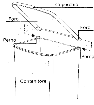
Figura B Montare il coperchio, forzando i due perni posti alle estremità posteriori del contenitore nei due fori laterali del coperchio.
